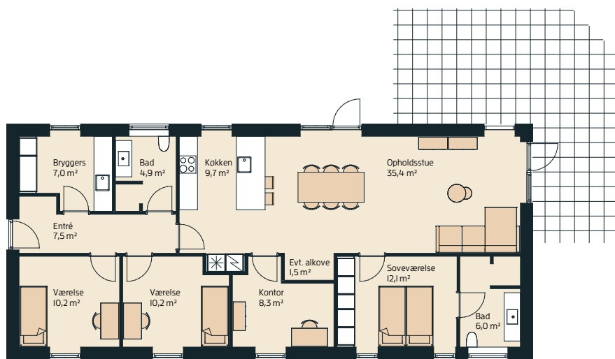
Længehus 137 m 2
