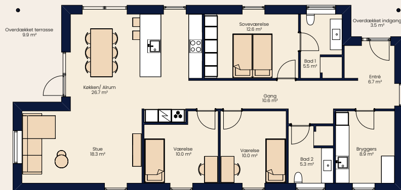
Længehus 140 m²
