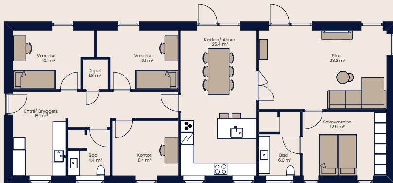
Længehus 146 m²
