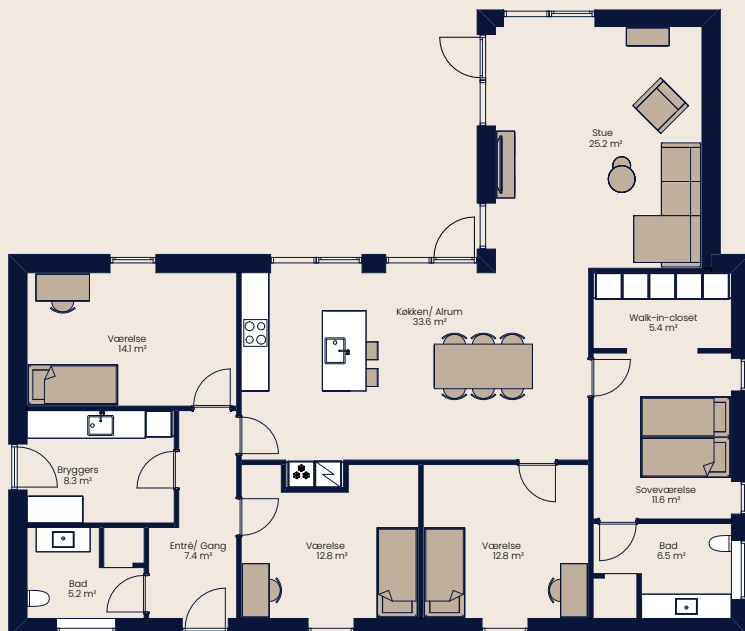
Vinkelhus 172 m²
