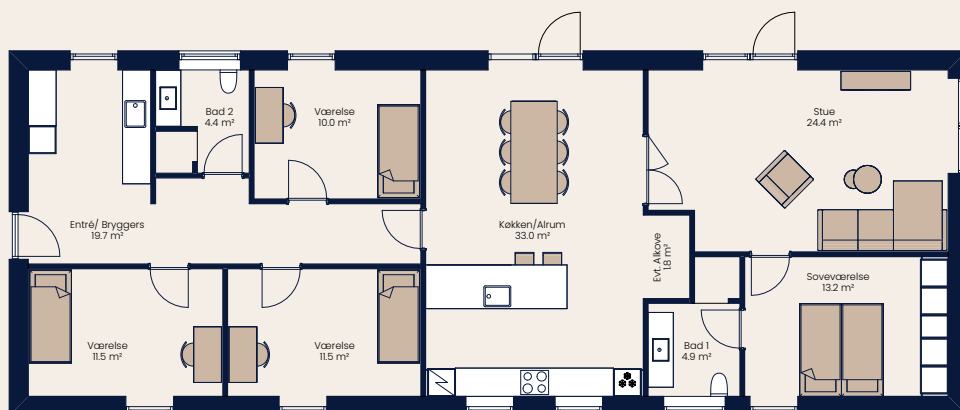
Længehus 162 m²
