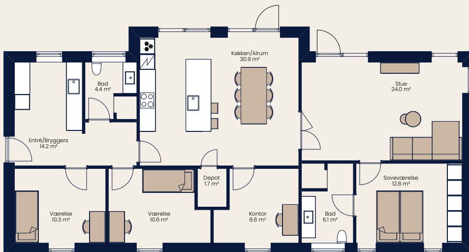
Vinkelhus 150 m²
