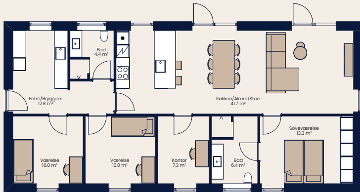
Længehus 129 m 2
