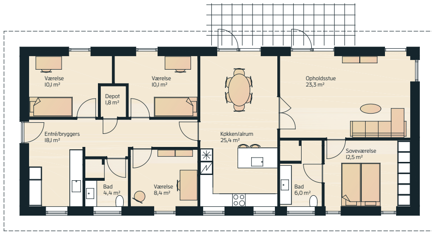
Længehus 146 m 2
