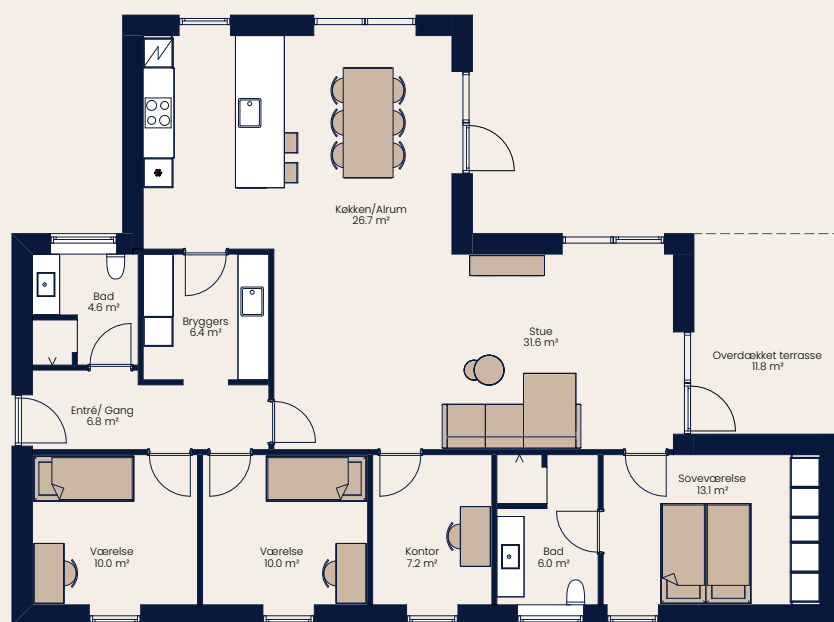
Vinkelhus 149 m 2
