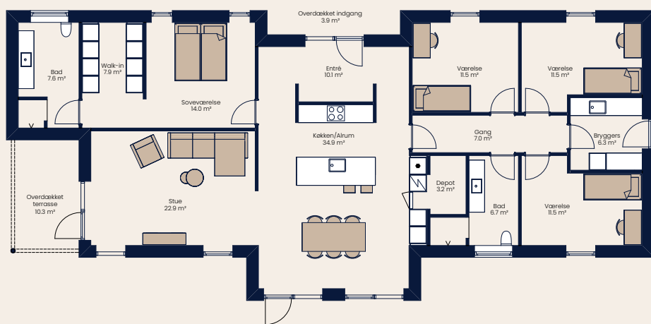
Vinkelhus 188 m 2
